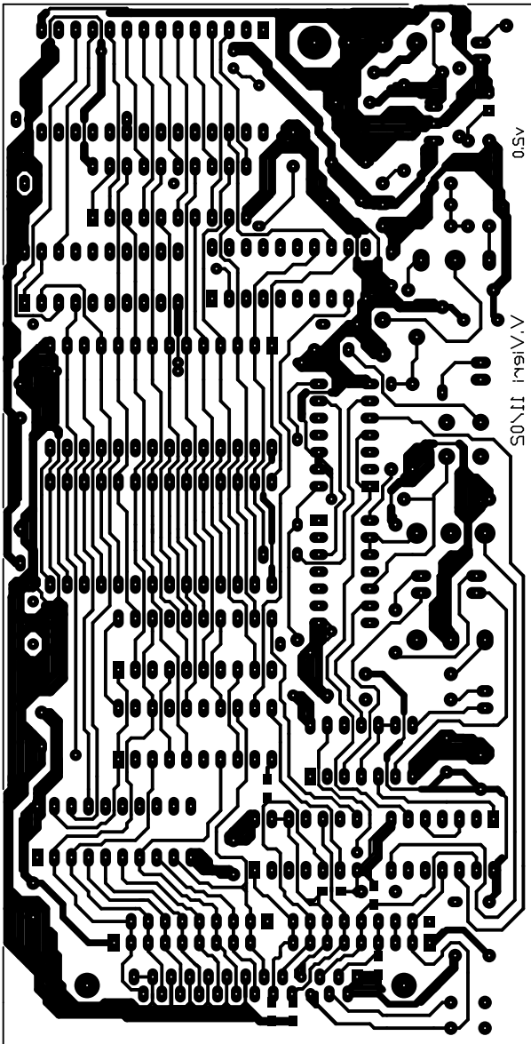
EPROM Bottom Layer
